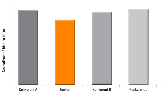
Porovnání hladiny hluku na základě výkonu konkurenčního výrobku s vůlí C3
